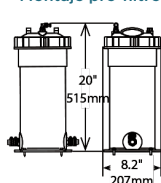
Montaje pre-filtro
