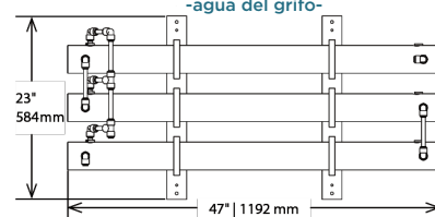
Montaje membrana -agua del grifo-
