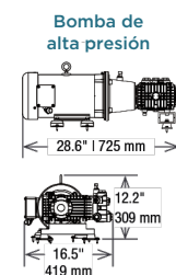
Bomba de alta presión
