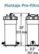
Montaje Pre-filtro
