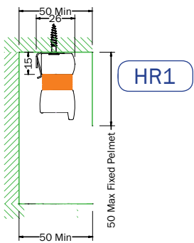
2 BAR RECESS FIXED BLIND Type: AO
