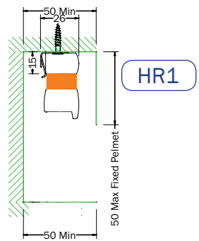
2 BAR RECESS FIXED BLIND Type: AO
